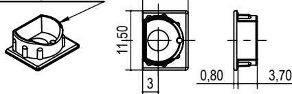
tappo per GN363 cover cap for GN363
